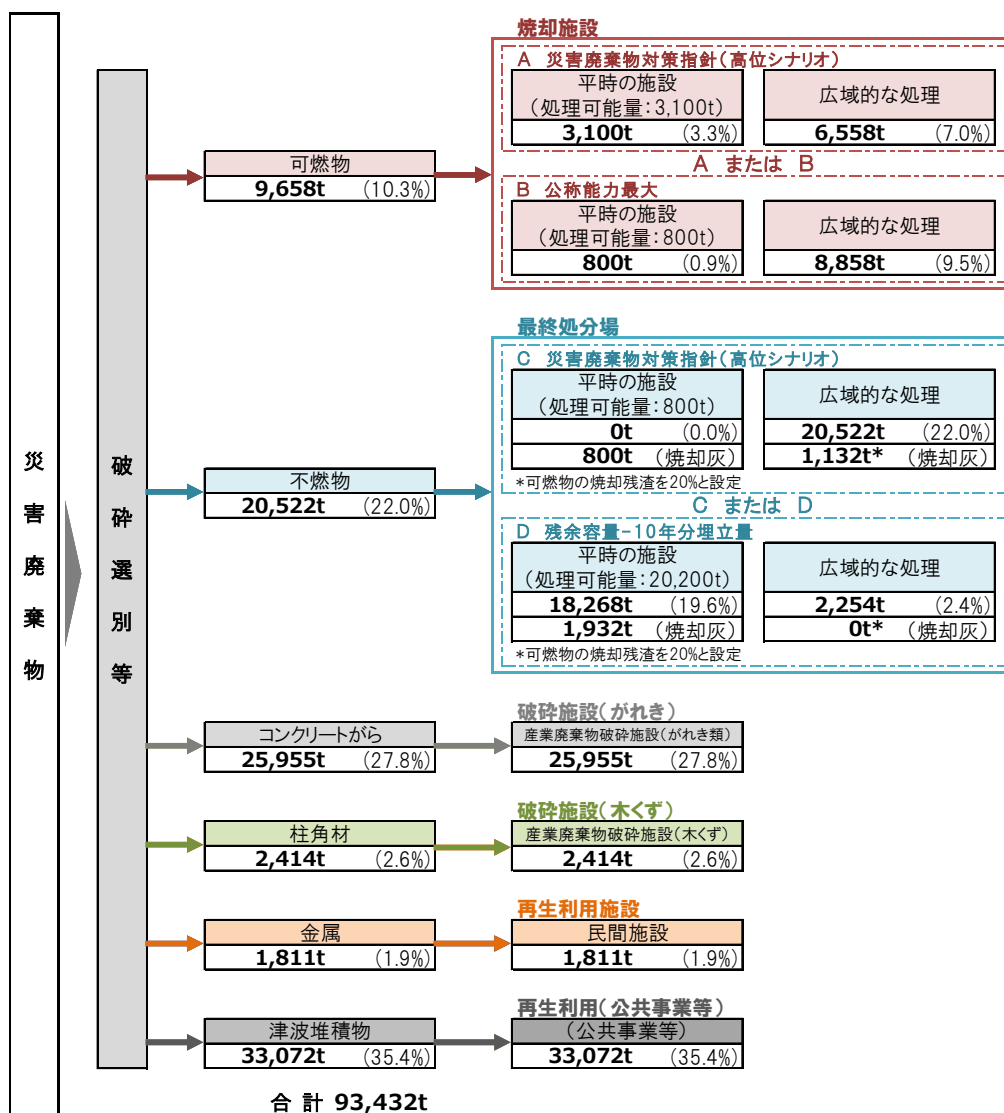
図9 種子島東方沖地震における災害廃棄物処理フロー
