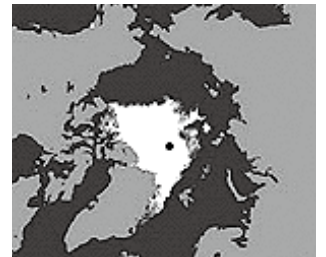
観測画像(平成24年の北極海海水の最小分布の様子)
