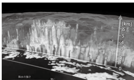
GPM主衛星が捉えた降水の3次元分布 (C)JAXA/NASA
