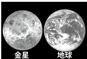
金星 地球 地球と金星は大きさと太陽からの距離が似ているが環境はまったく違う
