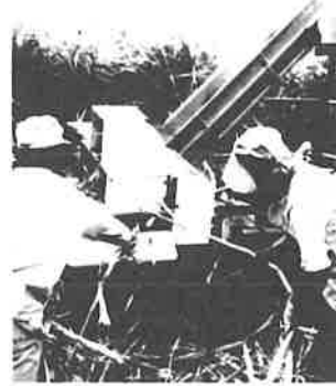
新しく導入したチョッピング式脱葉機で収穫する山根定之さん（満足山）
